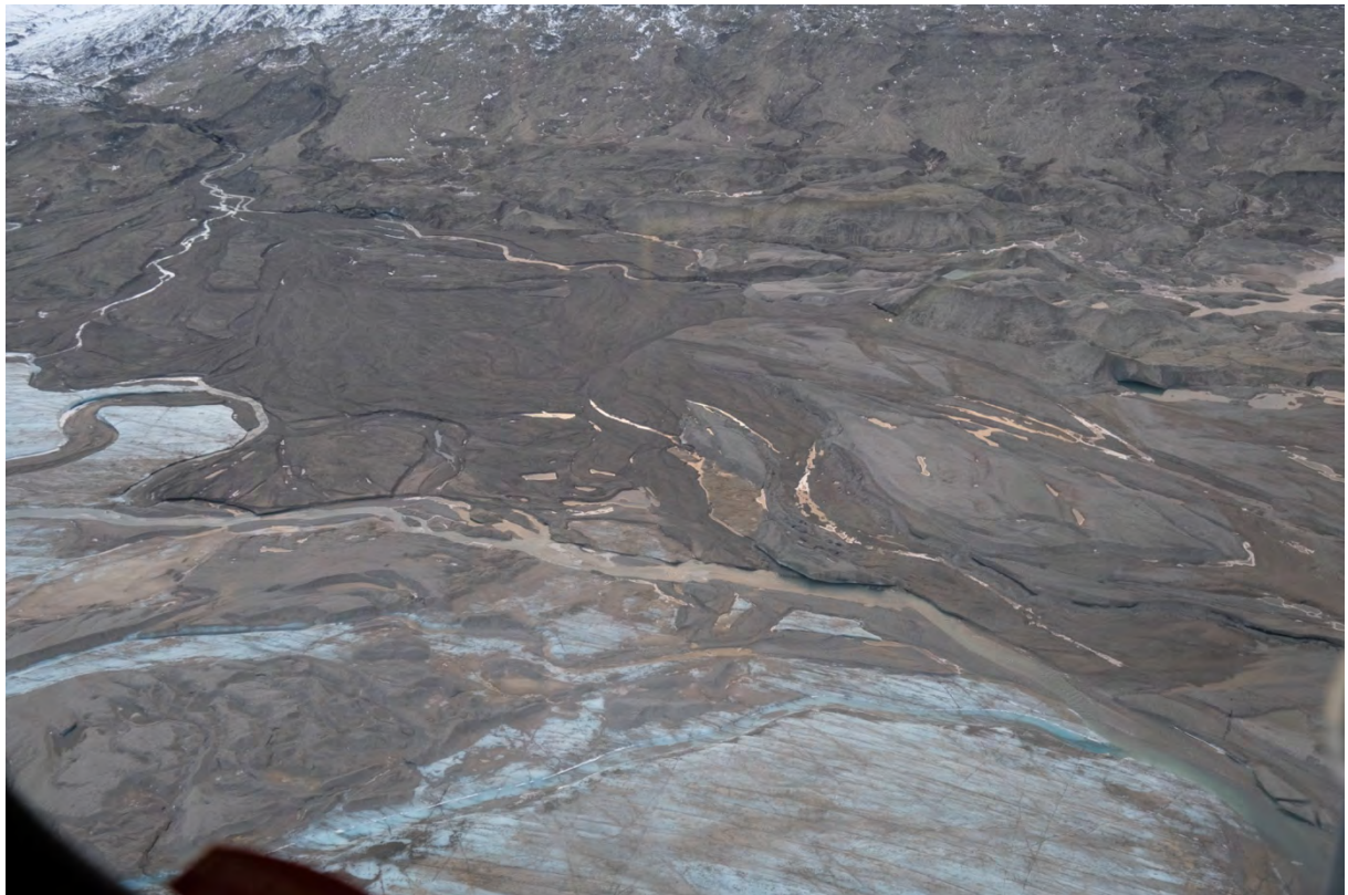
«Rasteplassen» i bunnen av Rabotbreen (bilde tatt mot sørøst)
