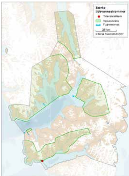
Figur 106: Sterke tidevannsstrømmer på Sentral-Spitsbergen. Akselsundet er markert.
